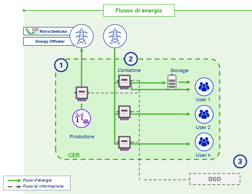
Figura 7 – Schematizzazione flussi energetici nel perimetro di una CER
