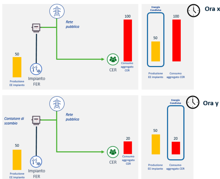
Figura 3 - Schema esemplificativo per il calcolo dell'energia condivisa
